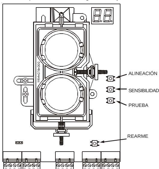
Figure 6: Ubicaciones de los botones
